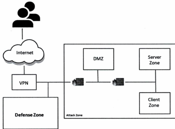
รูปภาพ Diagram : การแข่งขัน CTF Jeopardy ในรูปแบบ Attack the virtual World
