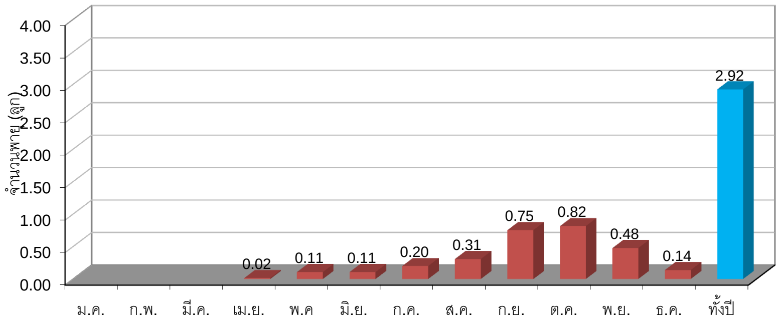
จำนวนพายุหมุนเขตร้อนเฉลี่ยที่เคลื่อนเข้าสู่ประเทศไทย
