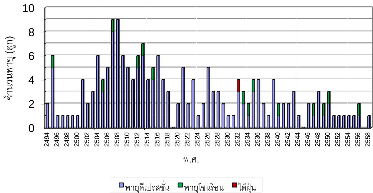
สถิติพายุหมุนเขตร้อนที่เคลื่อนเข้าสู่ประเทศไทย (พ.ศ.2494-2558)
