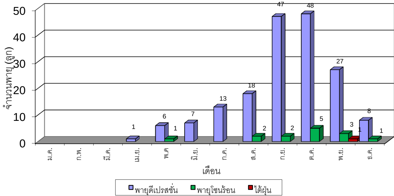
สถิติพายุหมุนเขตร้อนที่เคลื่อนเข้าสู่ประเทศไทย (พ.ศ.2494-2558)
