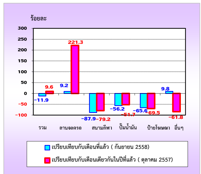
แผนภูมิ 3 เปรียบเทียบร้อยละของพื้นที่สิ่งก่อสร้างที่ได้รับอนุญาตให้ก่อสร้างใหม่ และต่อเติมดัดแปลงของสิ่งก่อสร้างที่มีใช้อาคารโรงเรียนทั่วประเทศ
