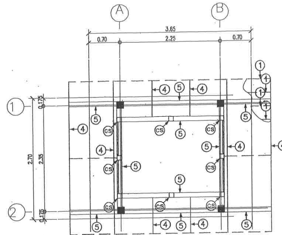
แปลนหลังคา(กลาง) SCALE 1:100
