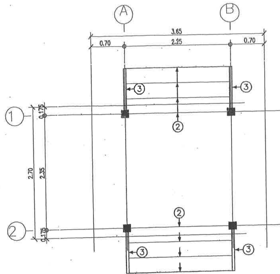
แปลนหลังคา(ล่าง) SCALE 1:100
