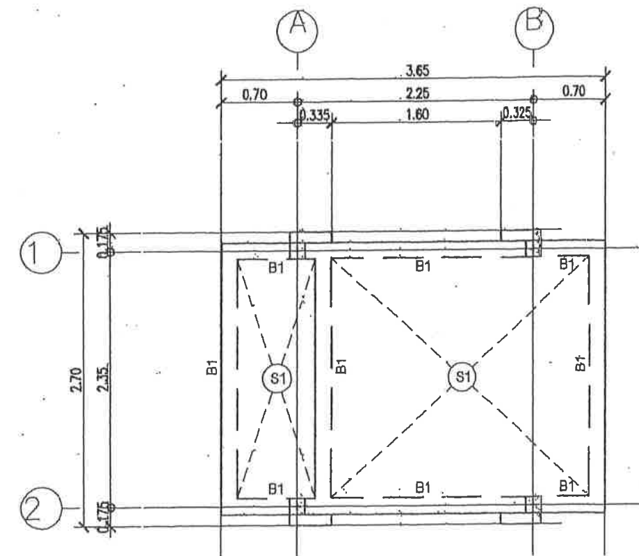
แปลนคานพื้นชั้น 1 SCALE 1:50
