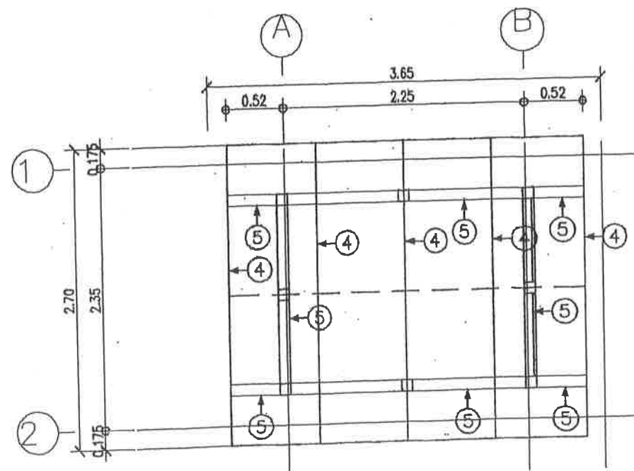
แปลนหลังคา(บน) SCALE 1:100
