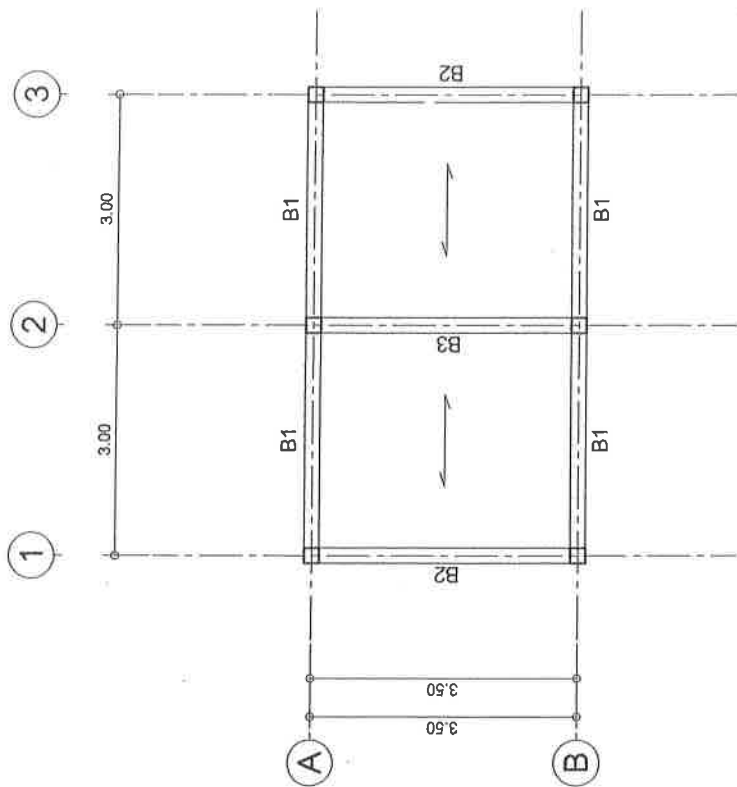
แปลนฐานราก มาตราส่วน 1:100
